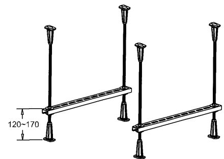
C SCALE 1:2
