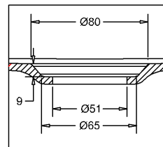
C SCALE 1:2
