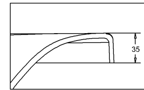
D SCALE 1:2
