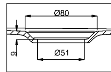
C SCALE 1:2
