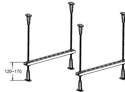
D SCALE 1:2
