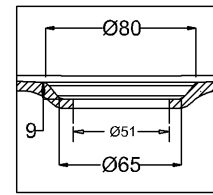
C SCALE 1:2
