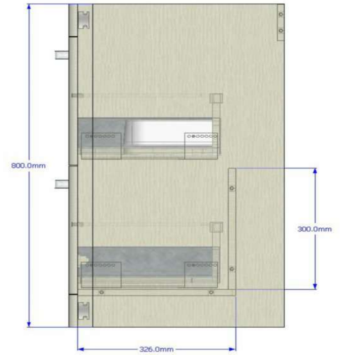
Right Elevation
